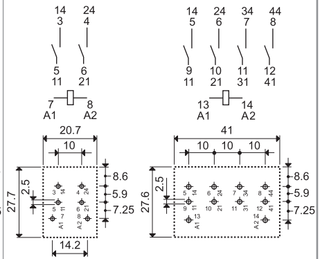
56.42-0300 Vue coté cuivre
