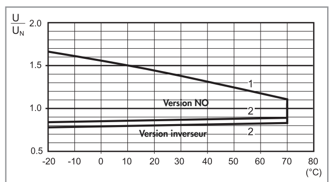
R 56 - Plage de fonctionnement bobine AC en fonction de la température ambiante, 4 inverseurs ou 4 NO
